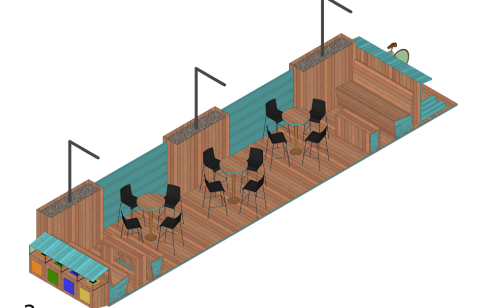
3 - PERGOLADO DE MADEIRA DE EUCALIPTO TRATADO
