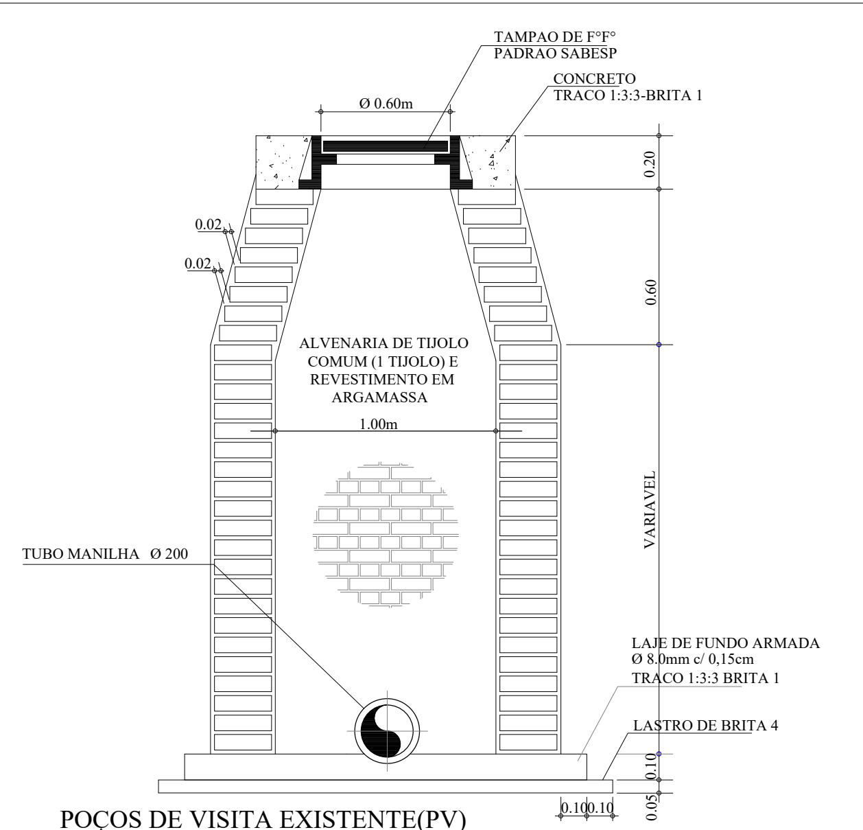
POÇOS DE VISITA EXISTENTE (PV) ESCALA 1:25
