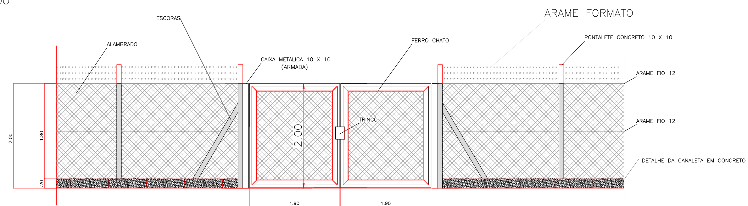
DETALHE DO PORTÃO ESCALA 1:50
