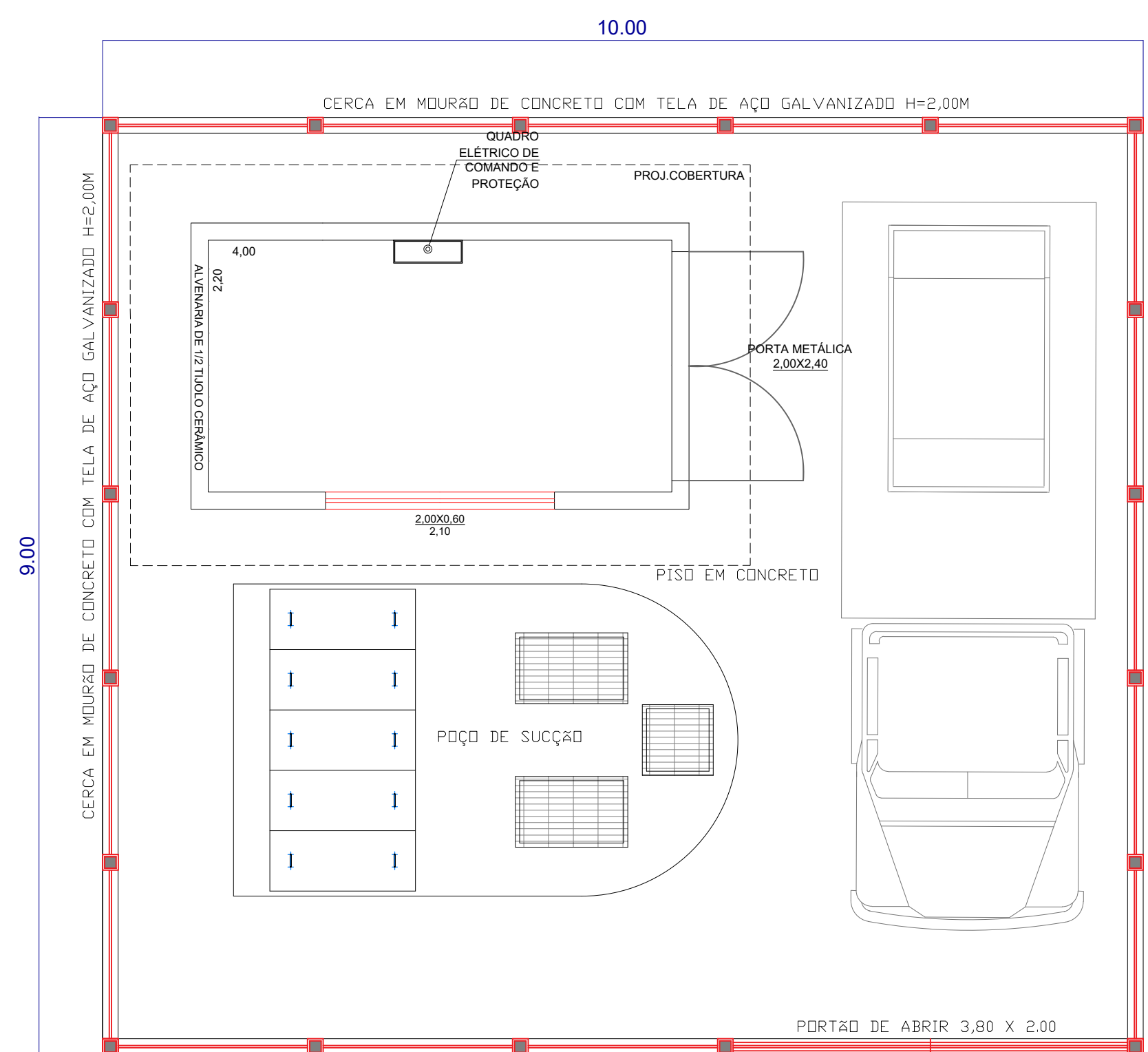
LAYOUT DE IMPLANTAÇÃO E.E.E (90,00 M2) ESCALA 1:50
